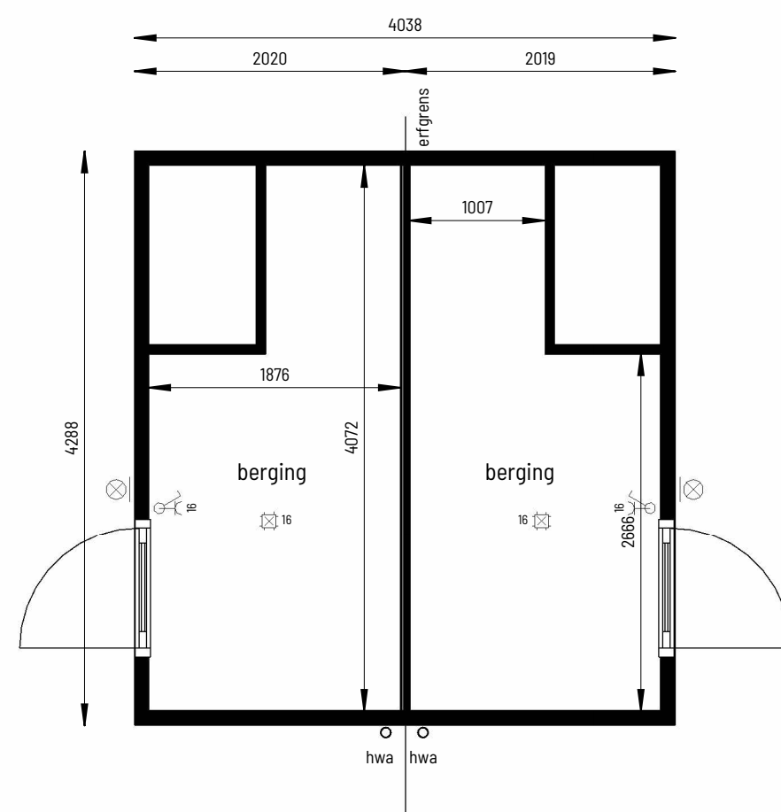
begane grond 1 : 50 - voor positie buitenbergingen zie situatietekening VK-00
